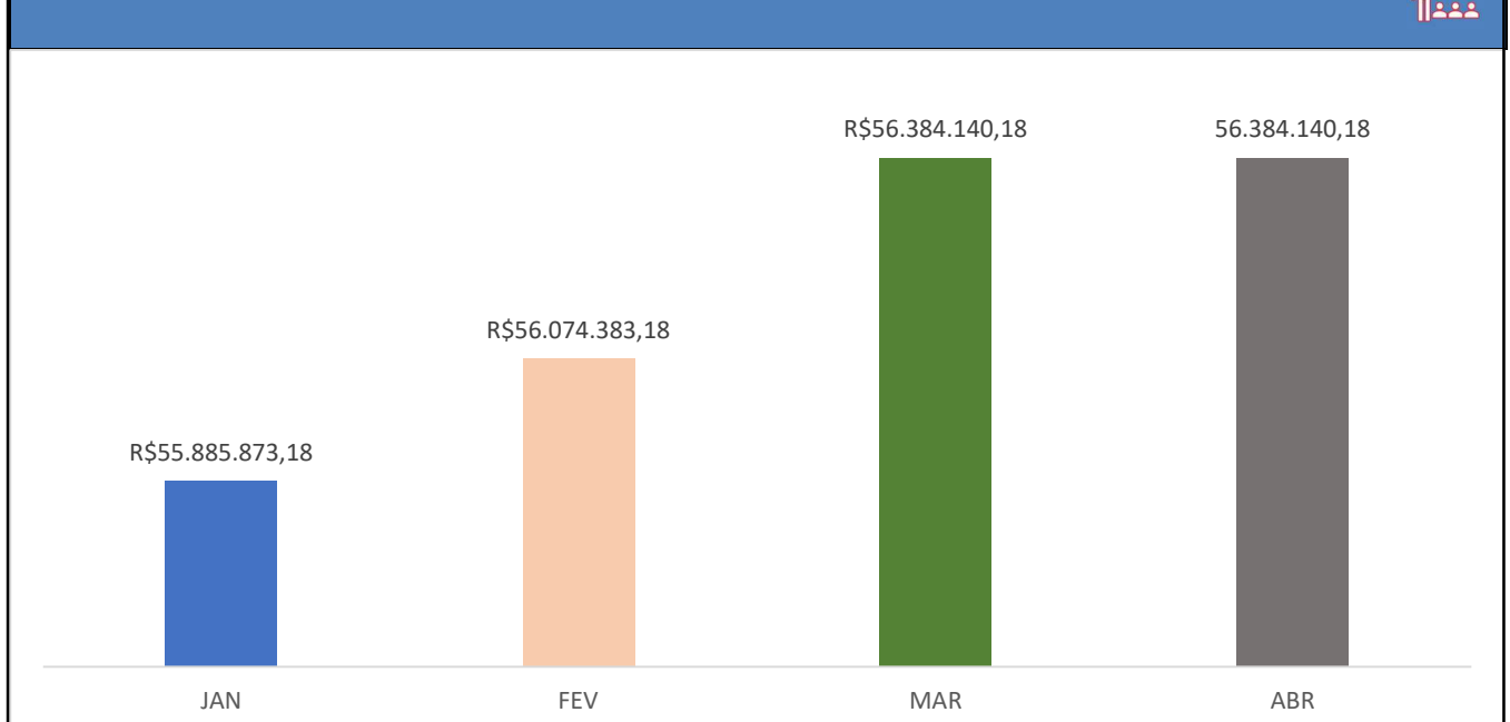
FIGURA 60: VALOR IMOBILIZADO
